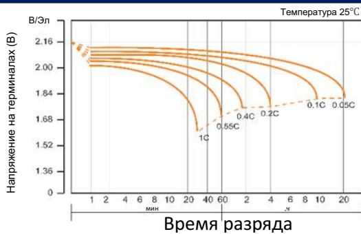
Кривые разряда
